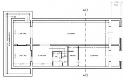
PIANTA PIANO INTERRATO
